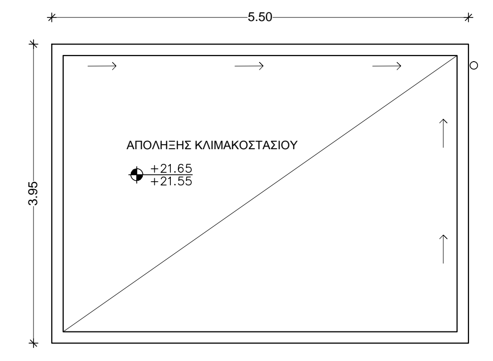
ΚΑΤΟΨΗ ΑΠΟΛΗΞΗΣ ΚΛΙΜΑΚΟΣΤΑΣΙΟΥ
